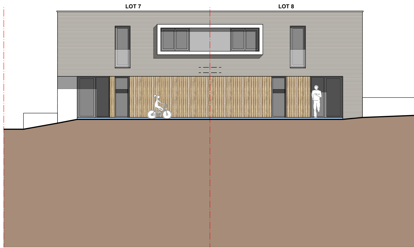
VORGEVEL 1/125
