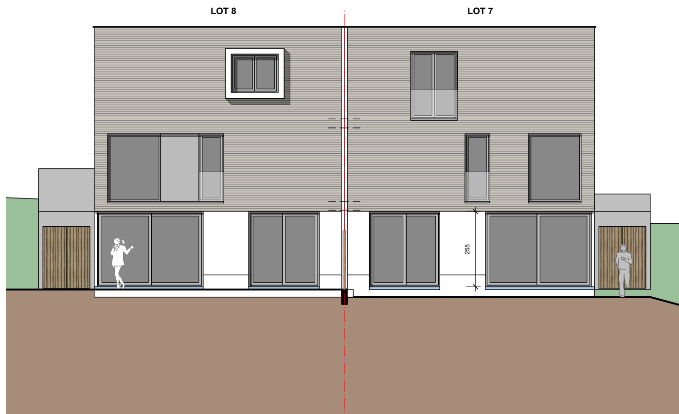
ACHTERGEVEL 1/125
