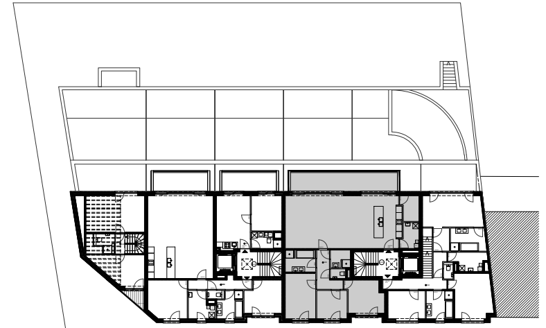
Grondplan 3de verdieping
